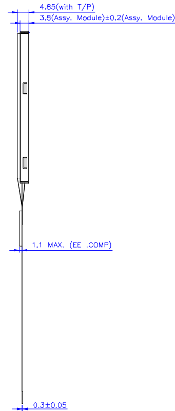
Outline Dimension of A040FL01 V2 Module
