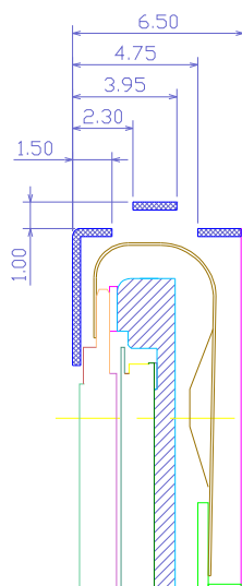
SECTION B-B(S:5/1)
