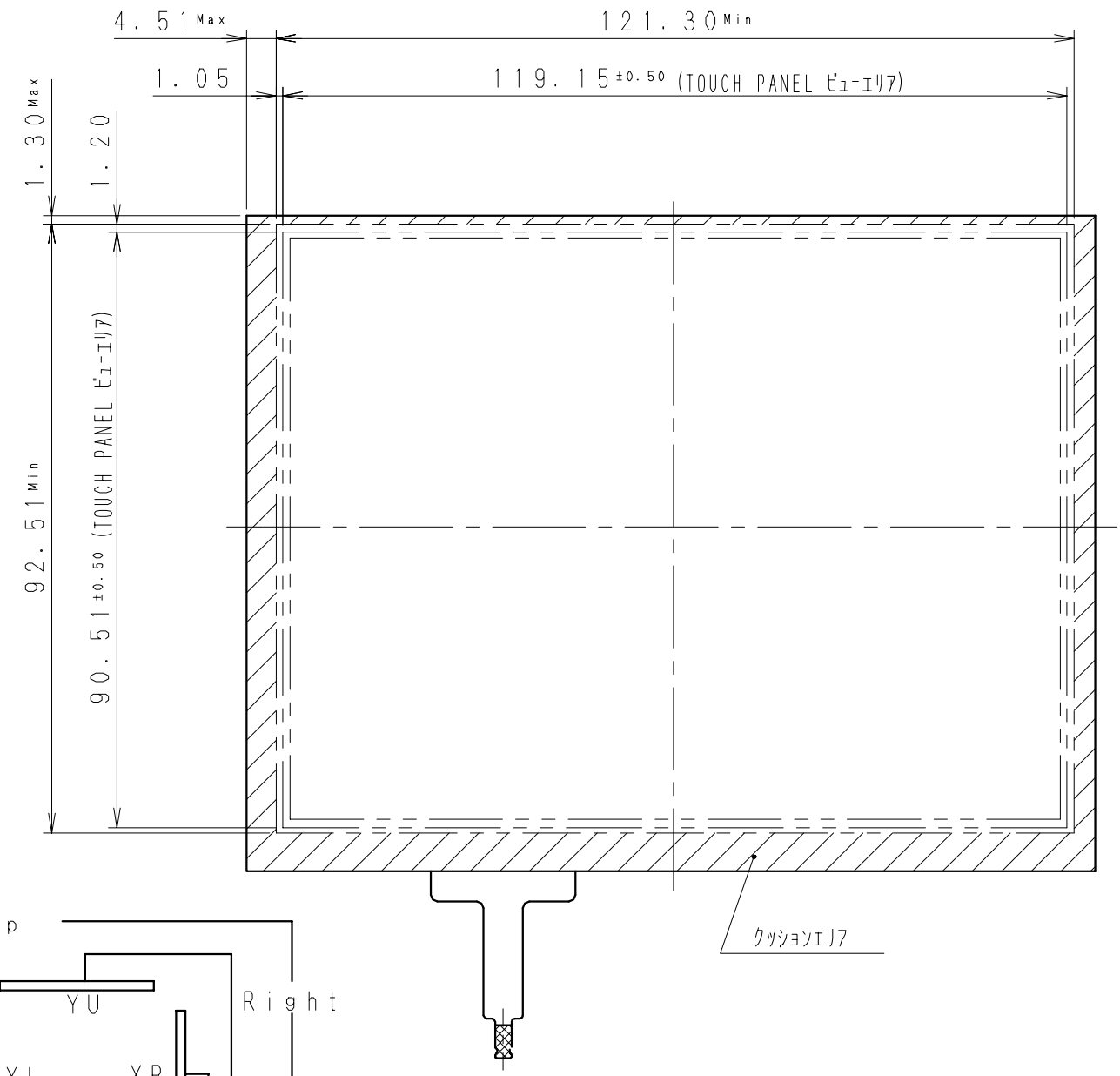
TOUCH PANEL クッションエリア (S=1/1)
