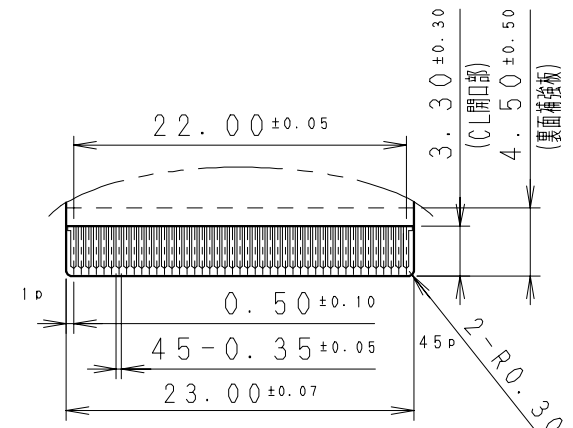
B部詳細図 (S=2/1)
