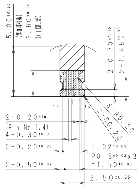
C部詳細図 (S=5/1)
