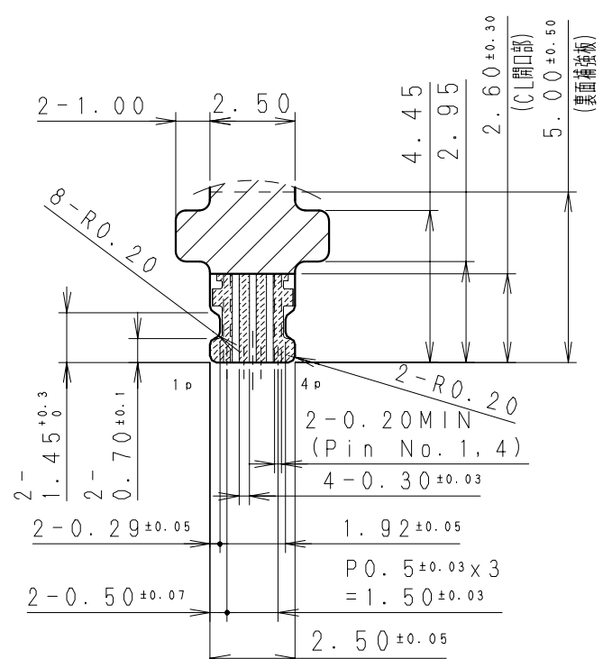
A部詳細図 (S=5/1)
