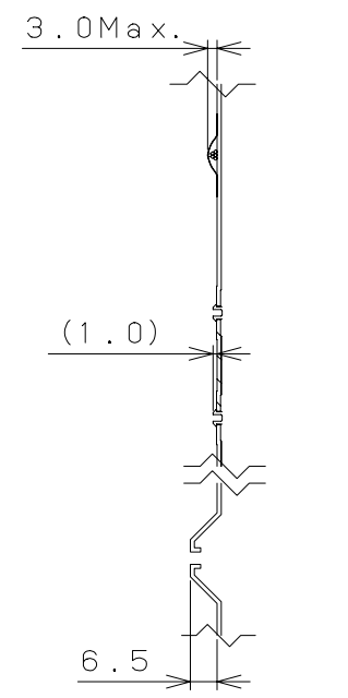
Section D-D
