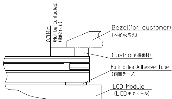
SECTION F-F(NTS)
