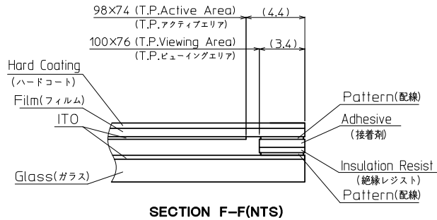
SECTION F-F(NTS)
