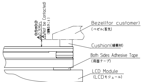
SECTION D-D(NTS)
