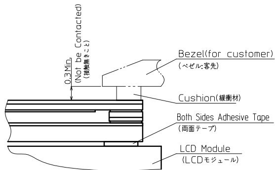
SECTION E-E(NTS)
