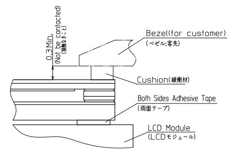
SECTION D-D(NTS)
