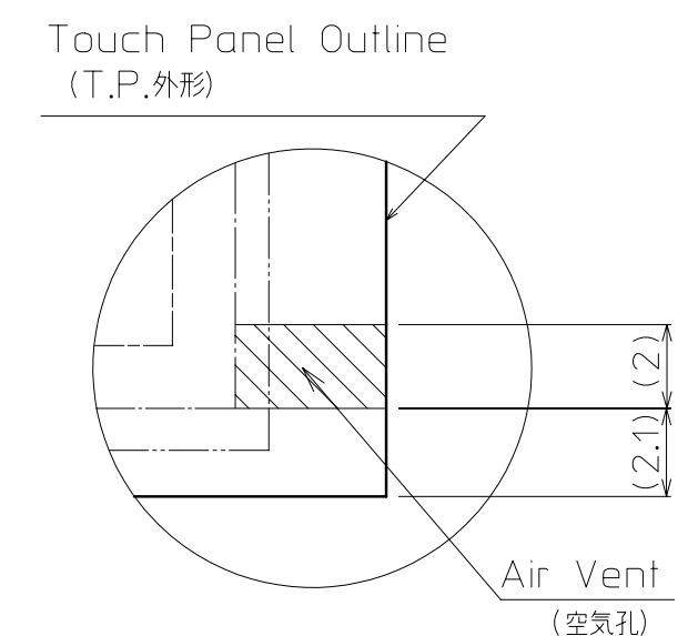
DETAIL C(5 : 1)
