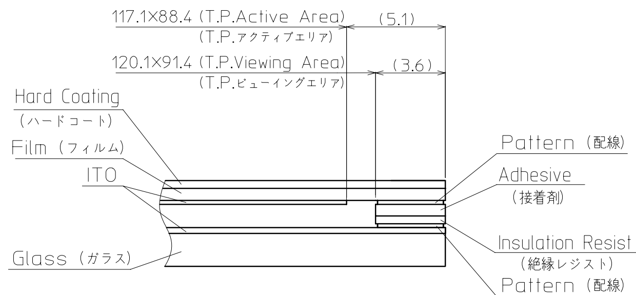
SECTION D-D(NTS)
