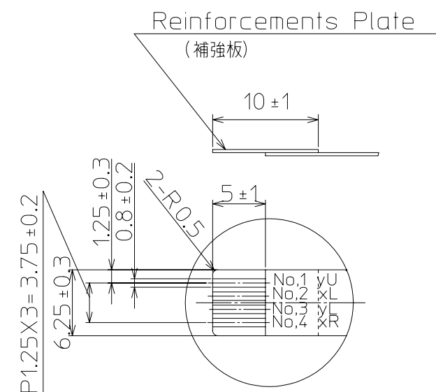
DETAIL B(2 : 1)
