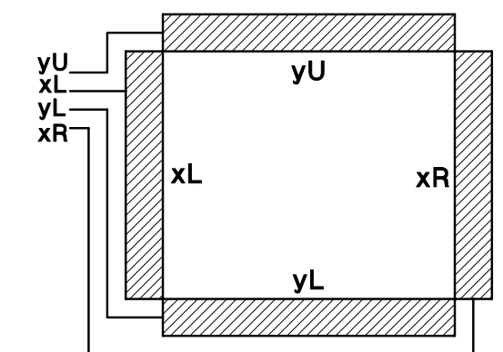
Touch Panel Pin-assign (タッチパネル ピンアサイン)
