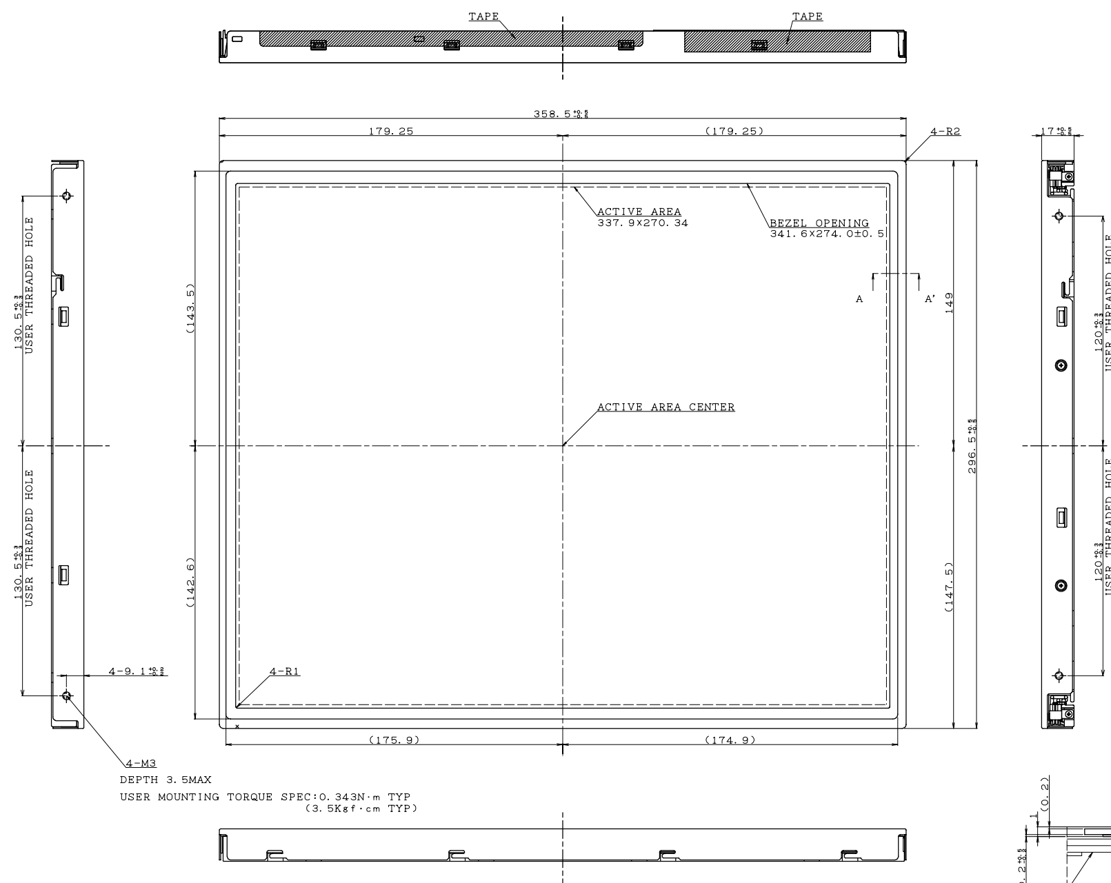
LQ170E1LG11 OUTLINE DIMENSIONS
